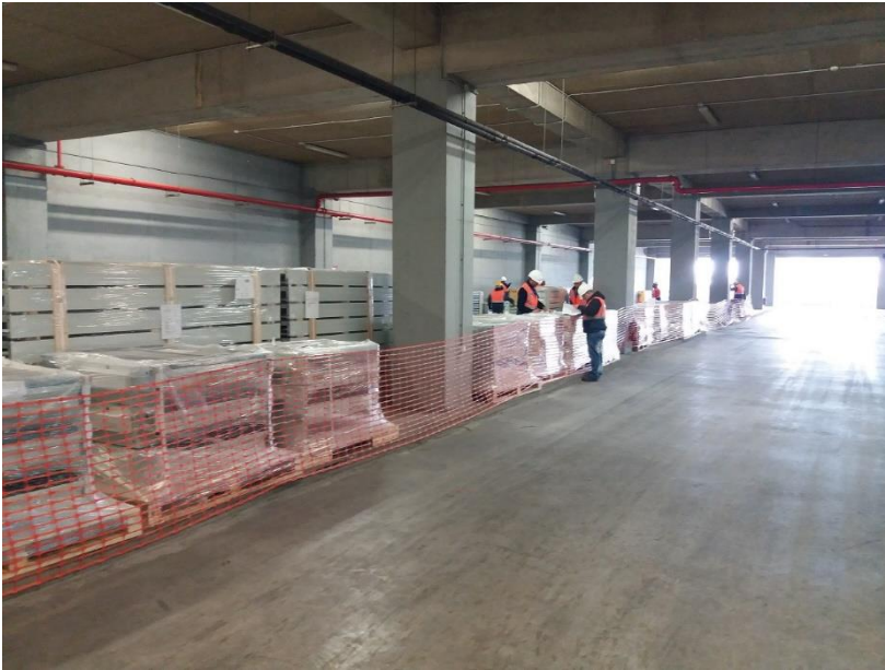
Παραλαβή εξαρτημάτων του νέου BHS – Delivery of BHS equipment
